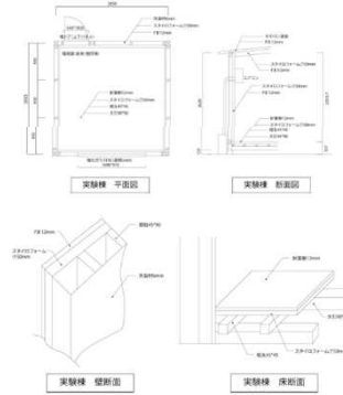
実験棟詳細
